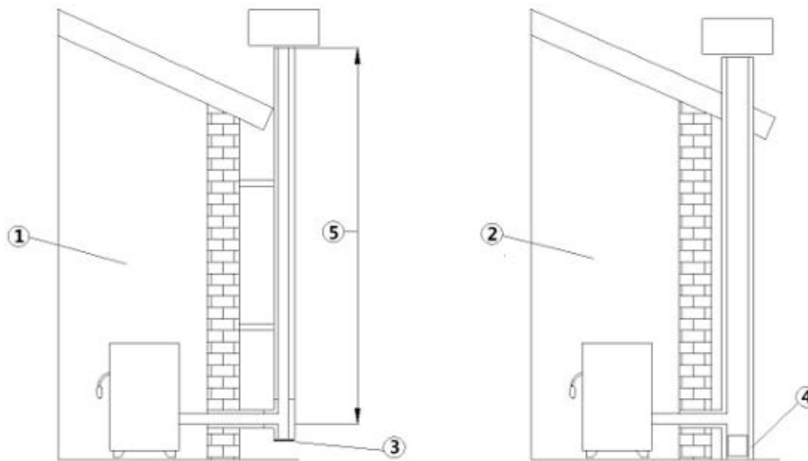
Fig. 1 - Rauchabzüge
