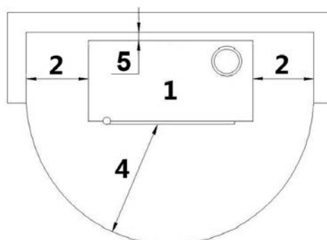
Fig. 56 - Wandinstallation
