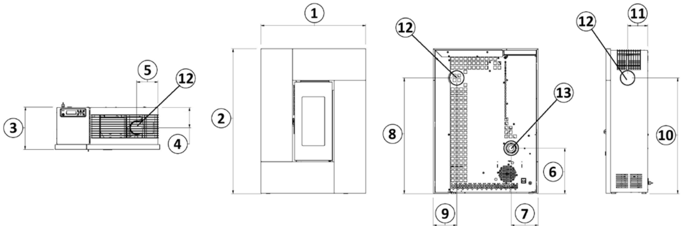
Fig. 13 - Allgemeine Abmessungen: Grace³
