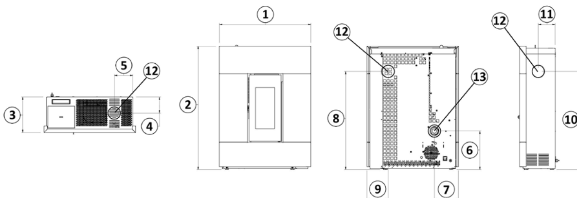
Fig. 17 - Allgemeine Abmessungen: Tabla
