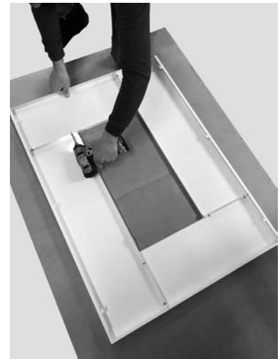
Fig. 24 - Befestigung der Platten 2
