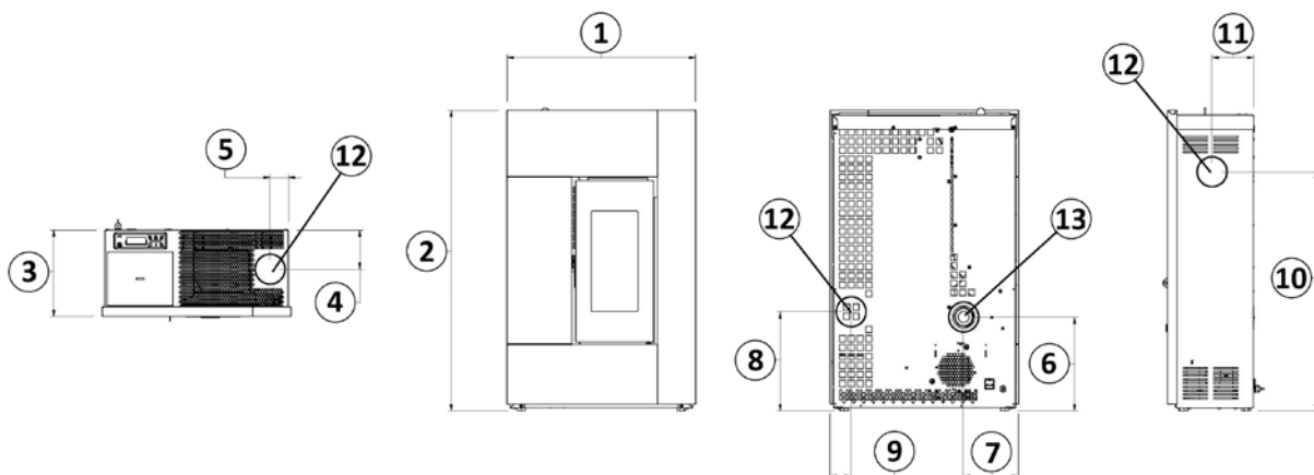
Fig. 12 - Allgemeine Abmessungen: Spirit 3
