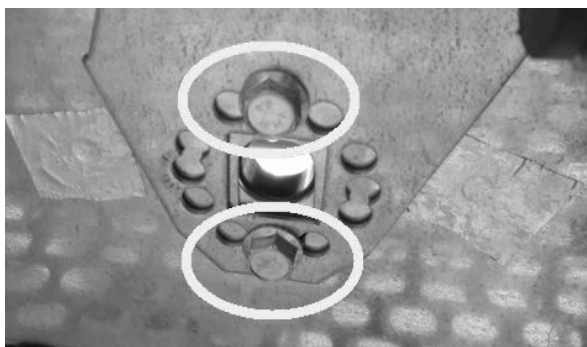
Fig. 73 - Die Schrauben entfernen
