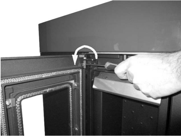
Fig. 20 - Entfernen der Schrauben
