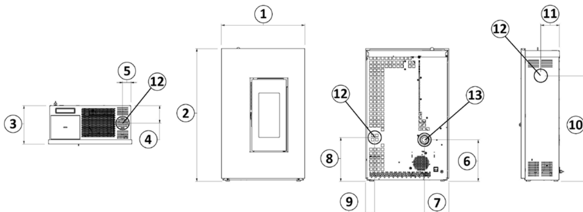
Fig. 16 - Allgemeine Abmessungen: Madison
