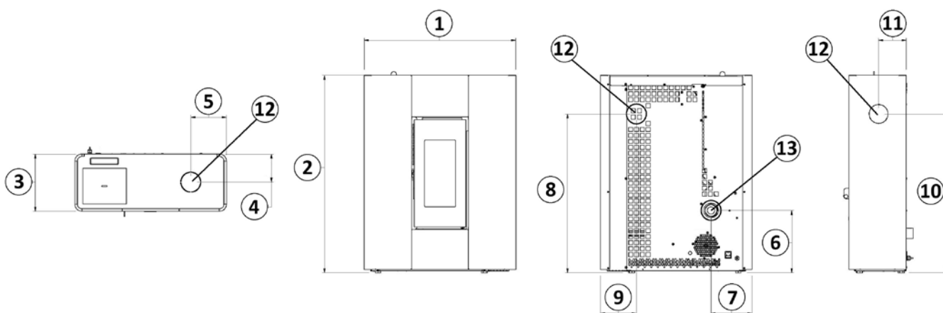
Fig. 15 - Allgemeine Abmessungen: Roxy
