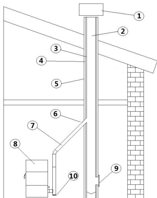
Fig. 5 - Bauteile Kamin
