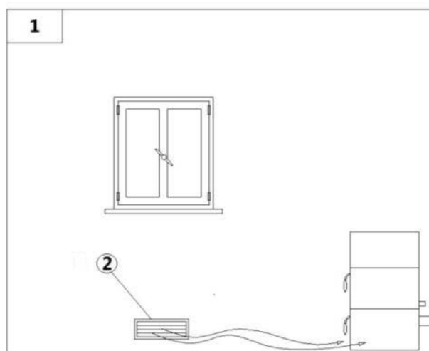
Fig. 9 - Direkte Luftzufuhr
