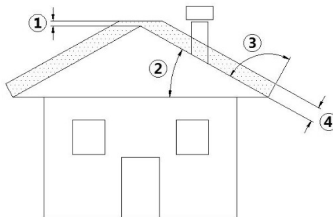
Fig. 2 - Geneigtes Dach
