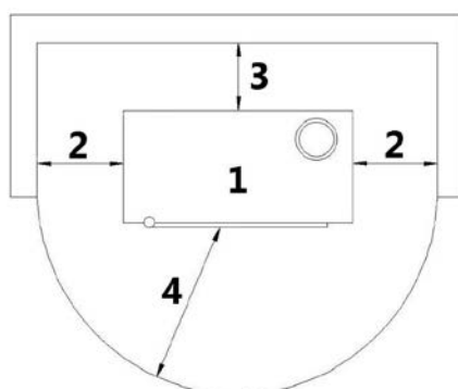
Fig. 19 - Allgemeine Installation
