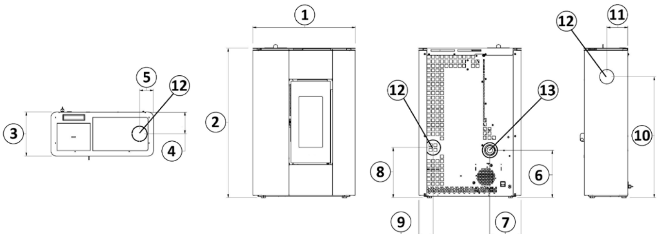
Fig. 14 - Allgemeine Abmessungen: Atrium
