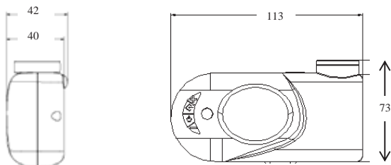
Zeichn. 1- Gehäuseabmessungen
